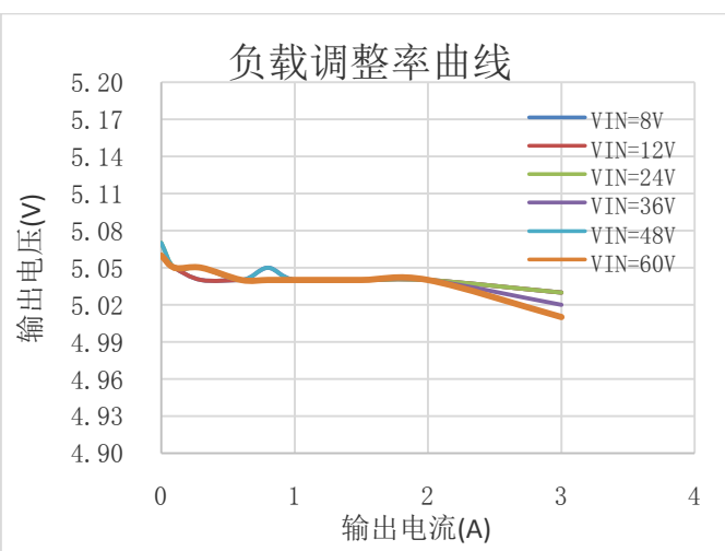
负载调整率
